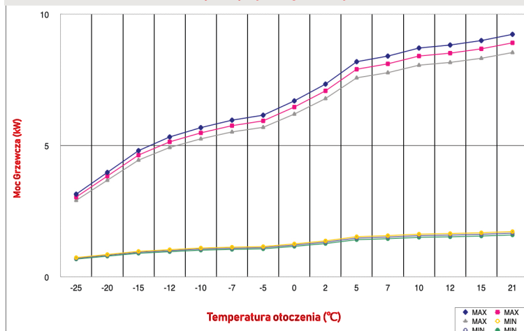
Krzywa wydajności grzewczej
