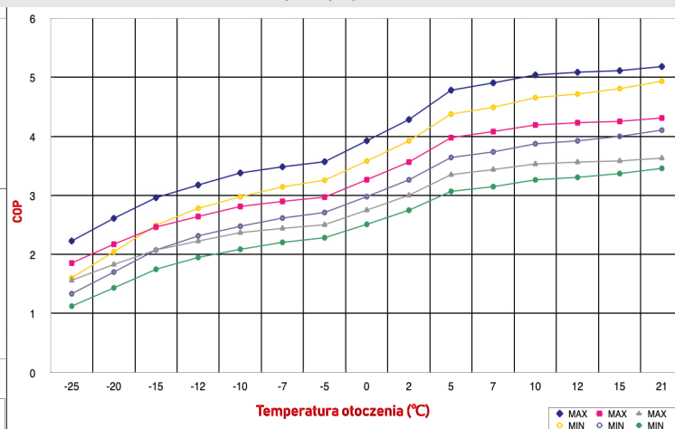
Krzywa wydajności COP
